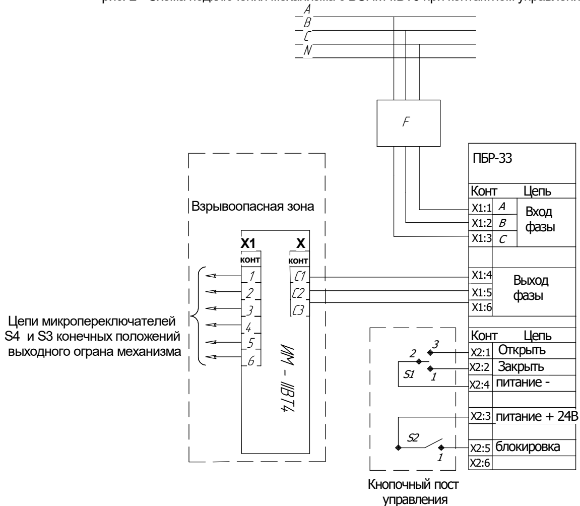
рис. 2 - Схема подключения механизма с БСПМ-ИВТ6 при контактном управлении
