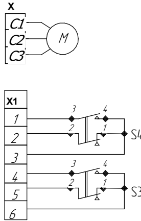
рис. 2 - Схема подключения механизма с БСПМ-ИВТ6 при контактном управлении
